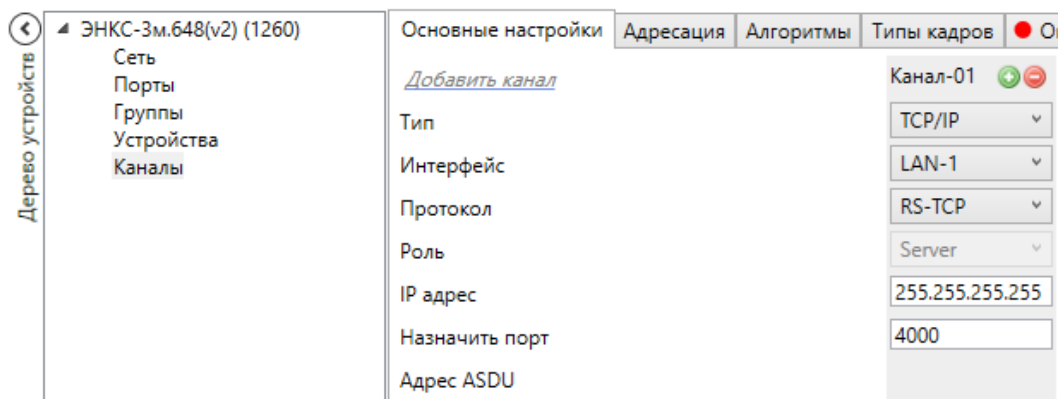
Рисунок 2.1. Настройка сквозного канала в ПО «ЭНКС Конфигуратор».
