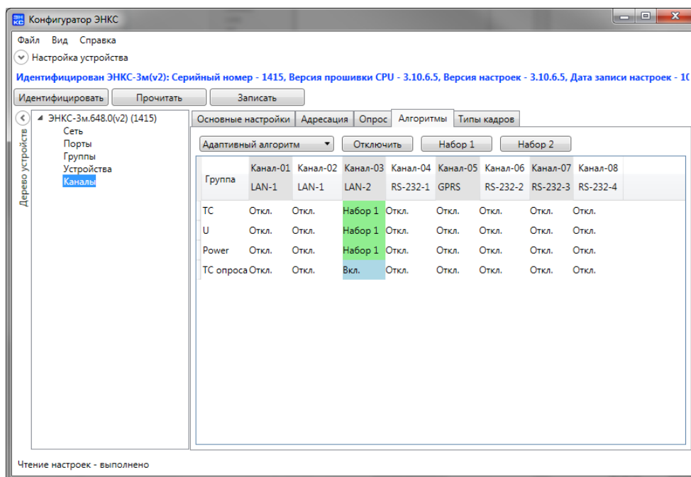
Рисунок 4.8. Включения передачи адаптивного алгоритма по одному из каналов.
