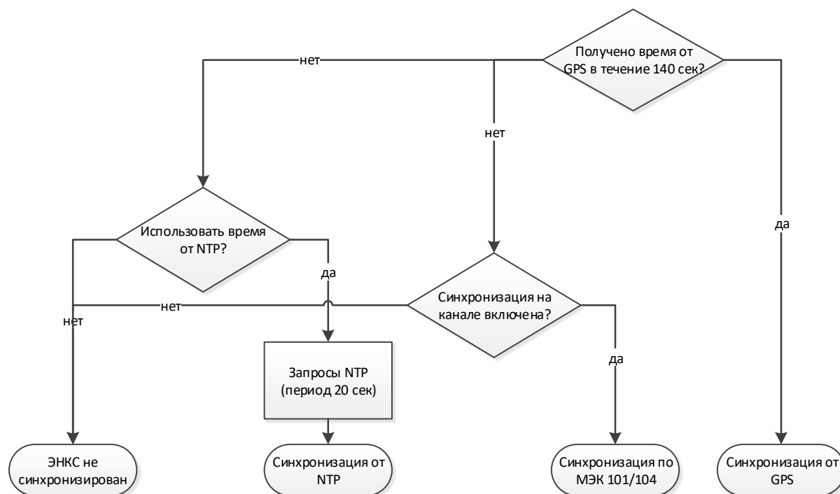
Рисунок 3.1. Алгоритм синхронизации внутренних часов в ЭНКС-3м.
