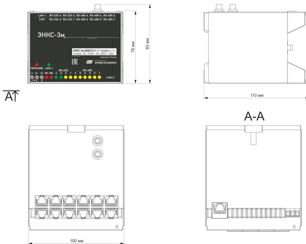
Рисунок 1.3. Габаритные размеры ЭНКС-3м.648GT-1.
