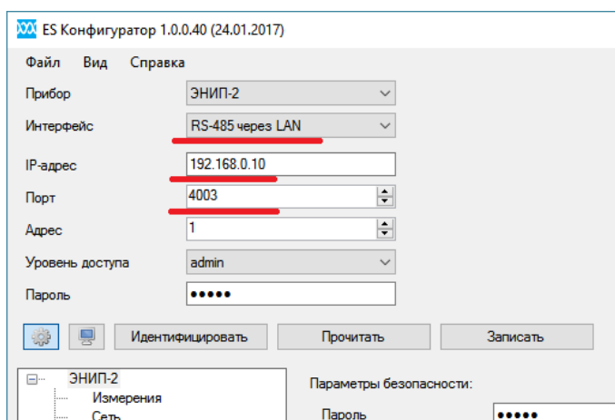
Рисунок 2.3. Пример настройки для подключения к ЭНИП-2 с использованием «сквозного канала», предоставляемого УСД ЭНКС-3м.
